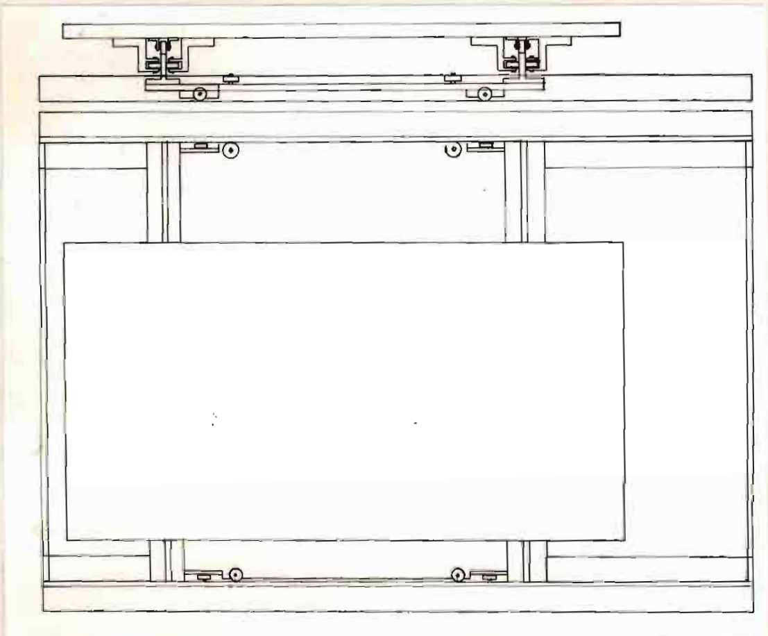
Fig. 12. Станок-штамп
